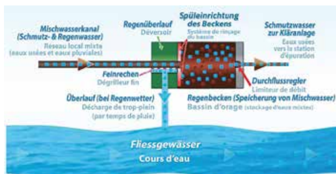
Funktionsprinzip eines Regenüberlaufbeckens
